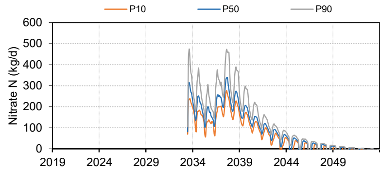
(d) Nitrate Load Reduction (kg/d)
